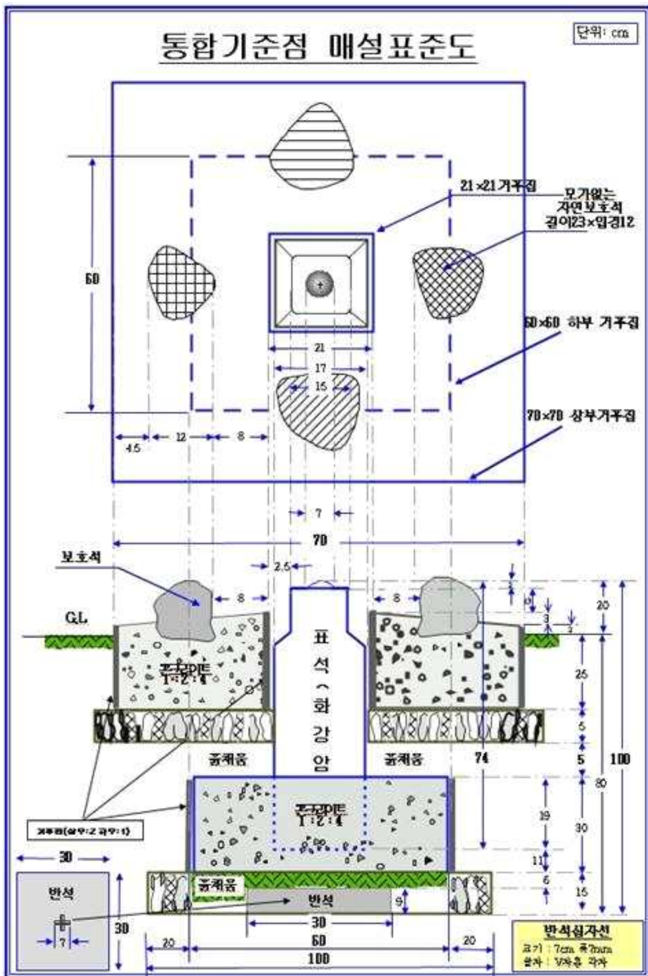
[별표 6-1] 통합기준점 매설표준도 (제17조제2항 관련)
